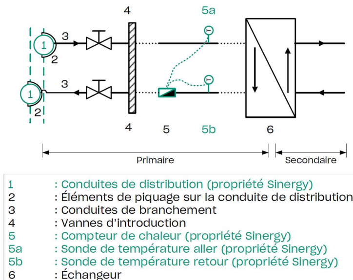
Figure 1 : Schéma limite de propriété FAD
